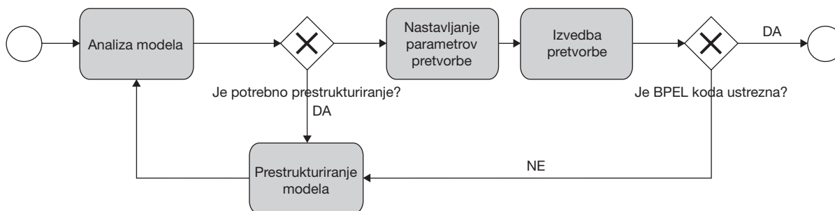
Slika 2: Postopek pretvorbe iz BPMN v BPEL
