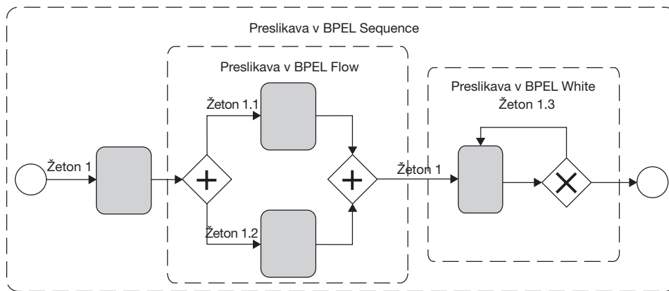
Slika 3: Primer statične tokovne analiza modela
