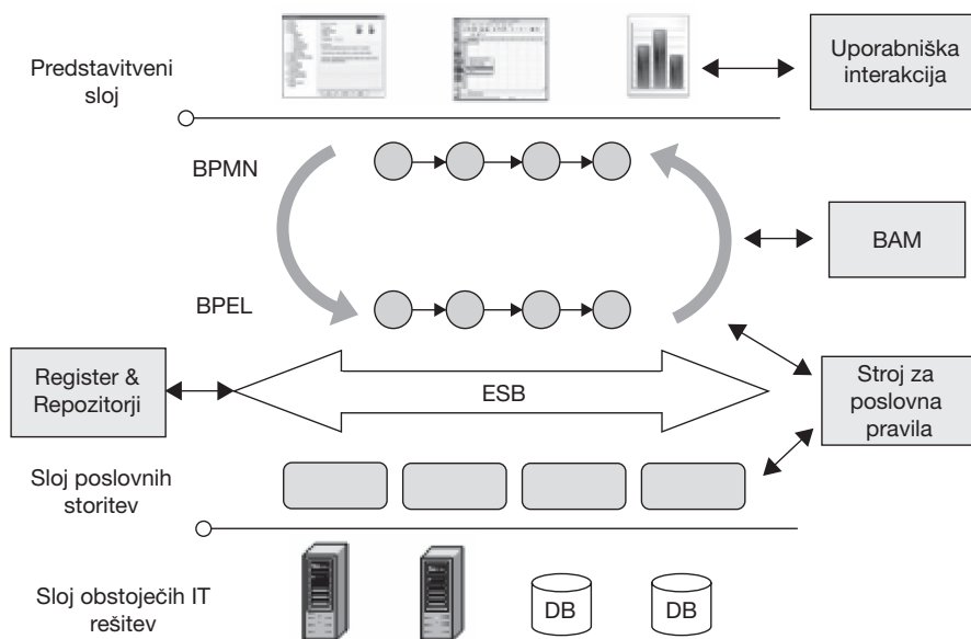
Slika 6: Arhitektura SOA
